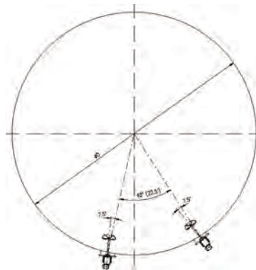
Obr. 1 – Schéma doporučeného uspořádání s bočními míchadly
